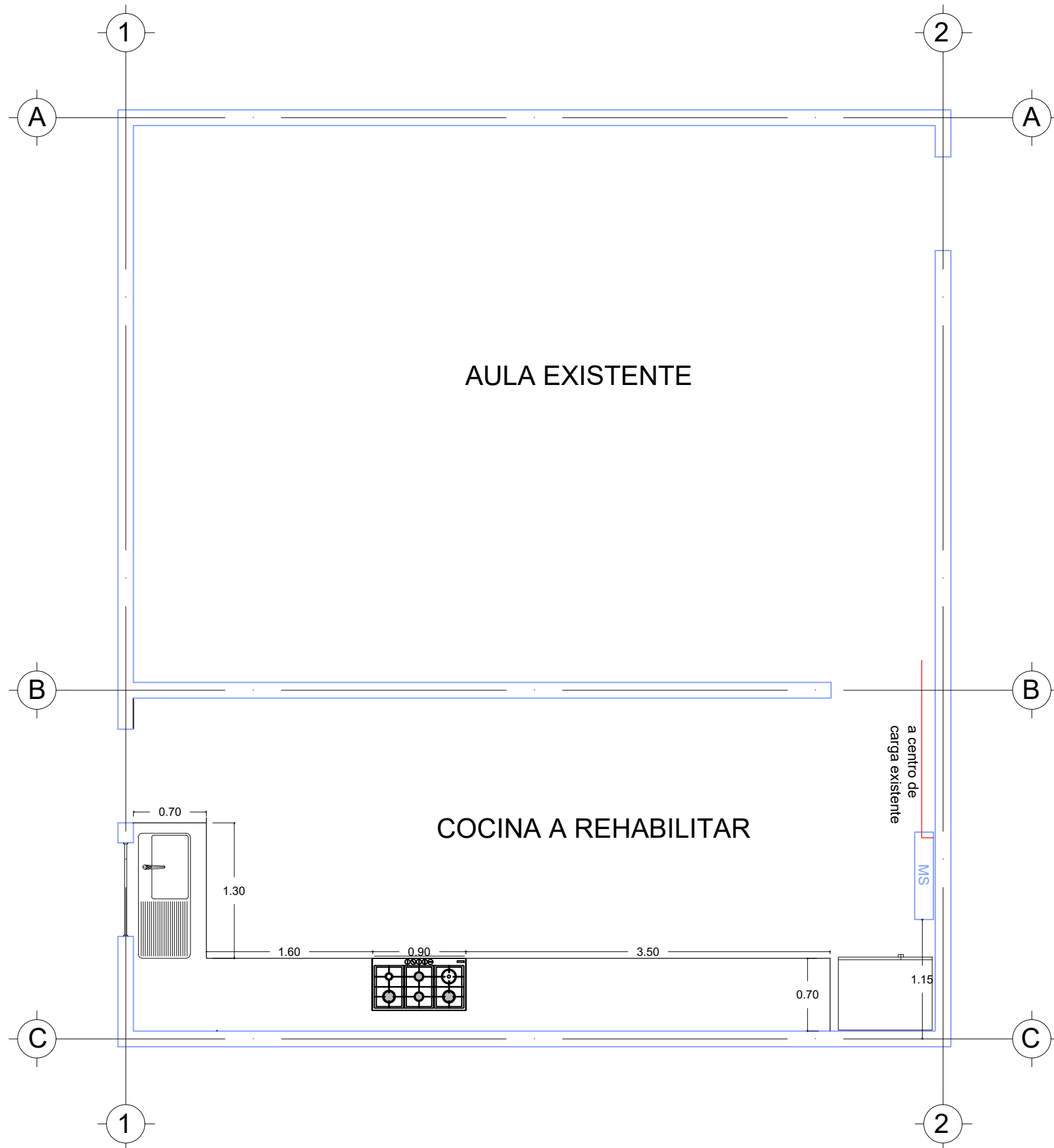
PLANTA ARQUITECTONICA
