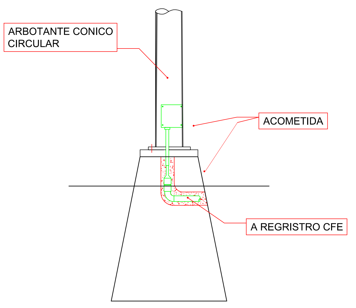
DETALLE ACOMETIDA
