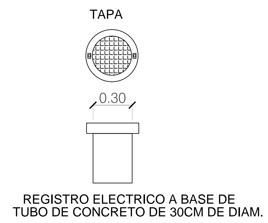
DETALLE REGISTRO ELECTRICO
