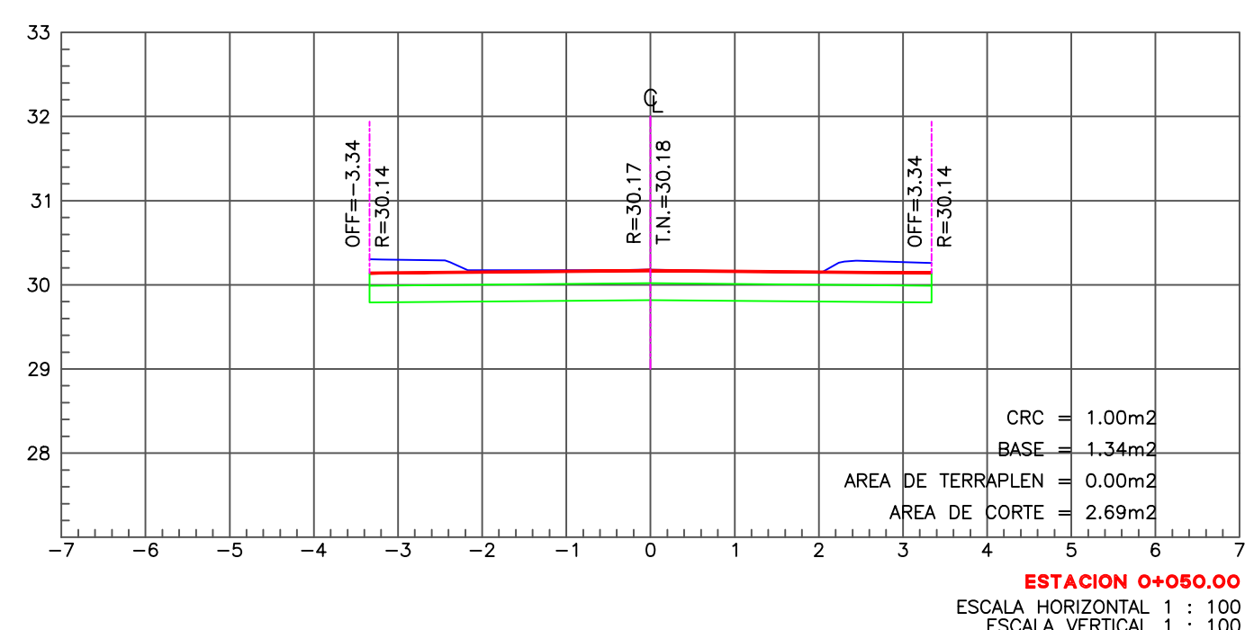
SECCIONES DE PROYECTO ESC. S/N
