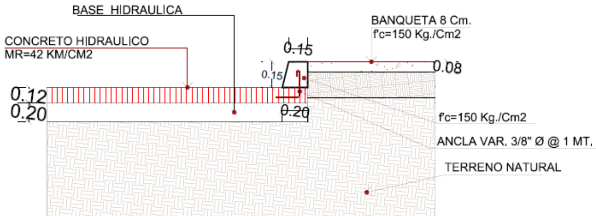
DETALLE DE GUARNICION TRAPEZOIDAL
