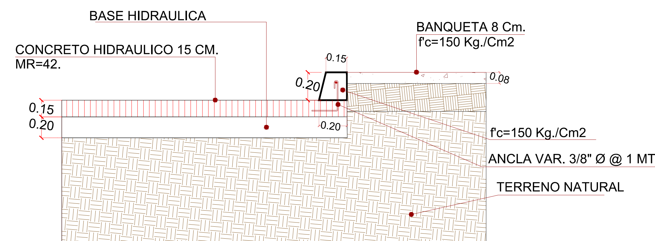
DETALLE DE GUARNICION TRAPEZOIDAL
