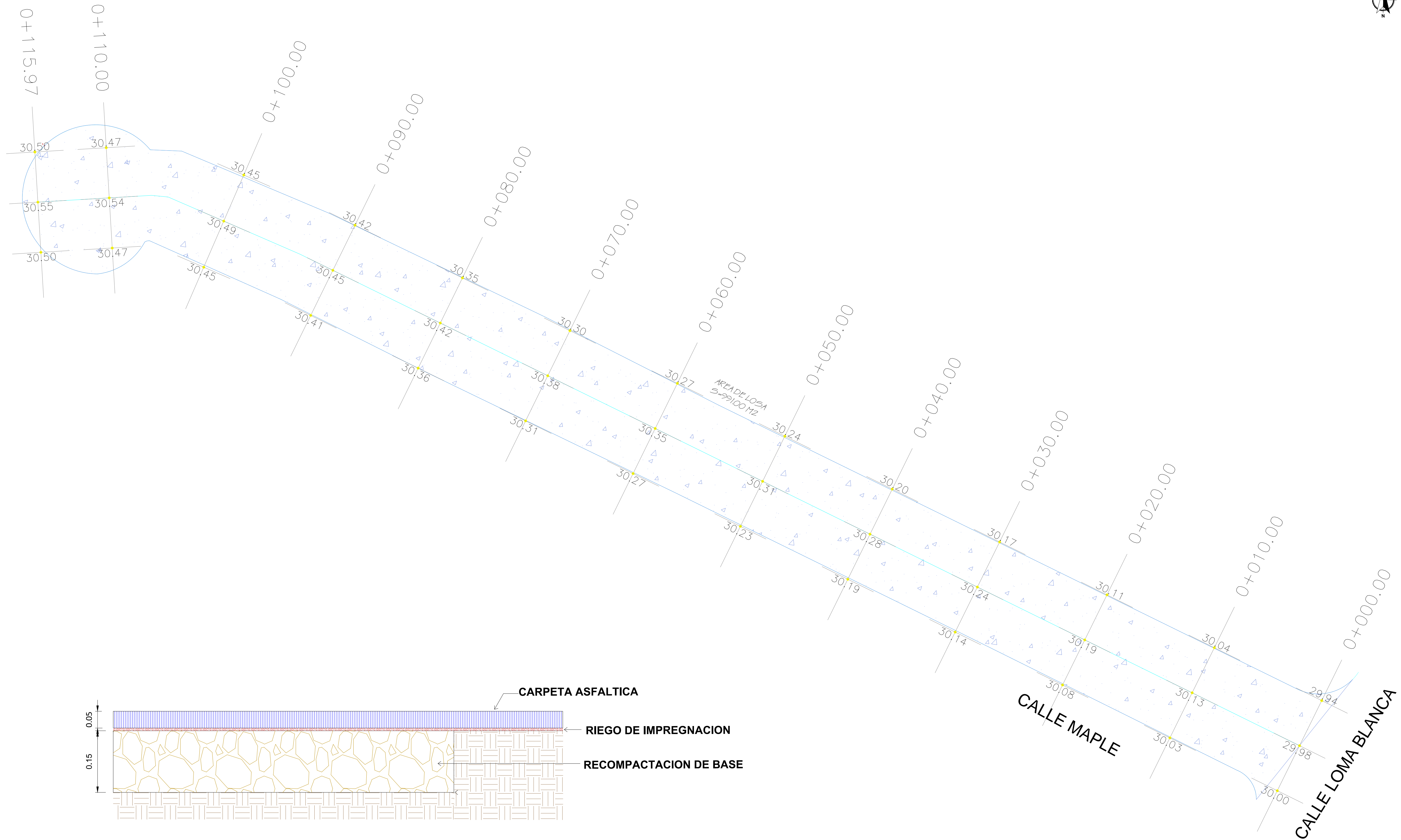
PLANTA GEOMETRICA CALLE MAPLE ESC: S/E
